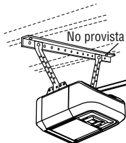
(No provista) Tornillos para madera de 5/16 de pulg. -18 x 1-7/8 de pulg.
